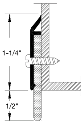
WT-323 Door Bottom Sweep Black Neoprene
