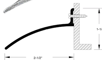
WT-R201 Door Top Rain Drip
